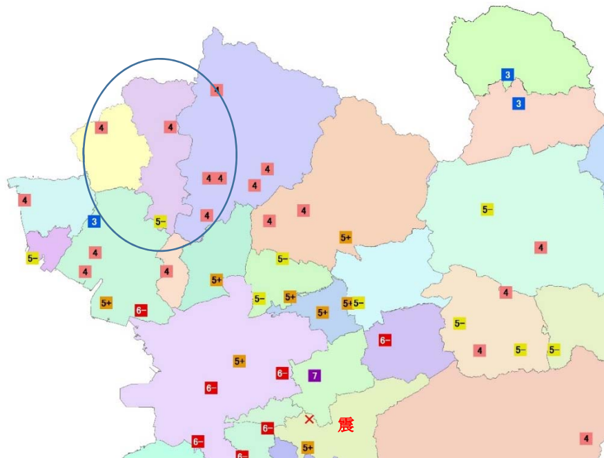
図 熊本地震(4月14日 21:26 発生 マグニチュード 6.5)における和水平町の震度
