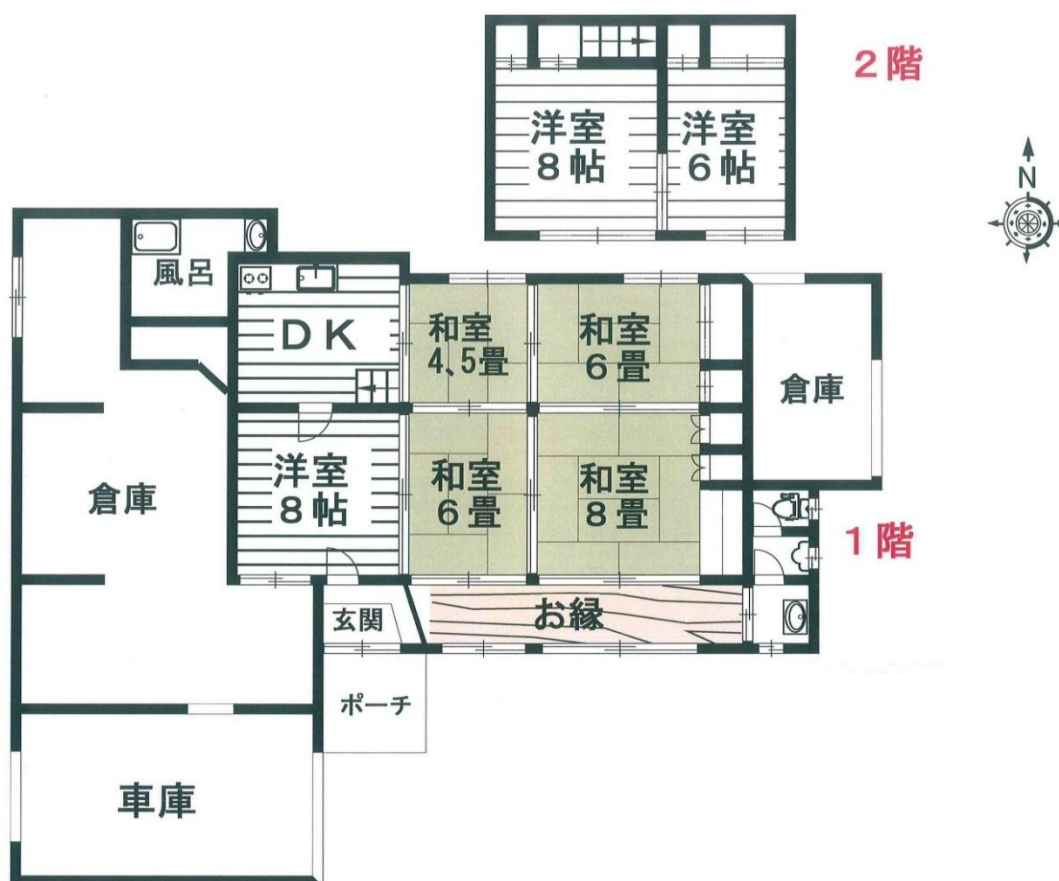
間取図
