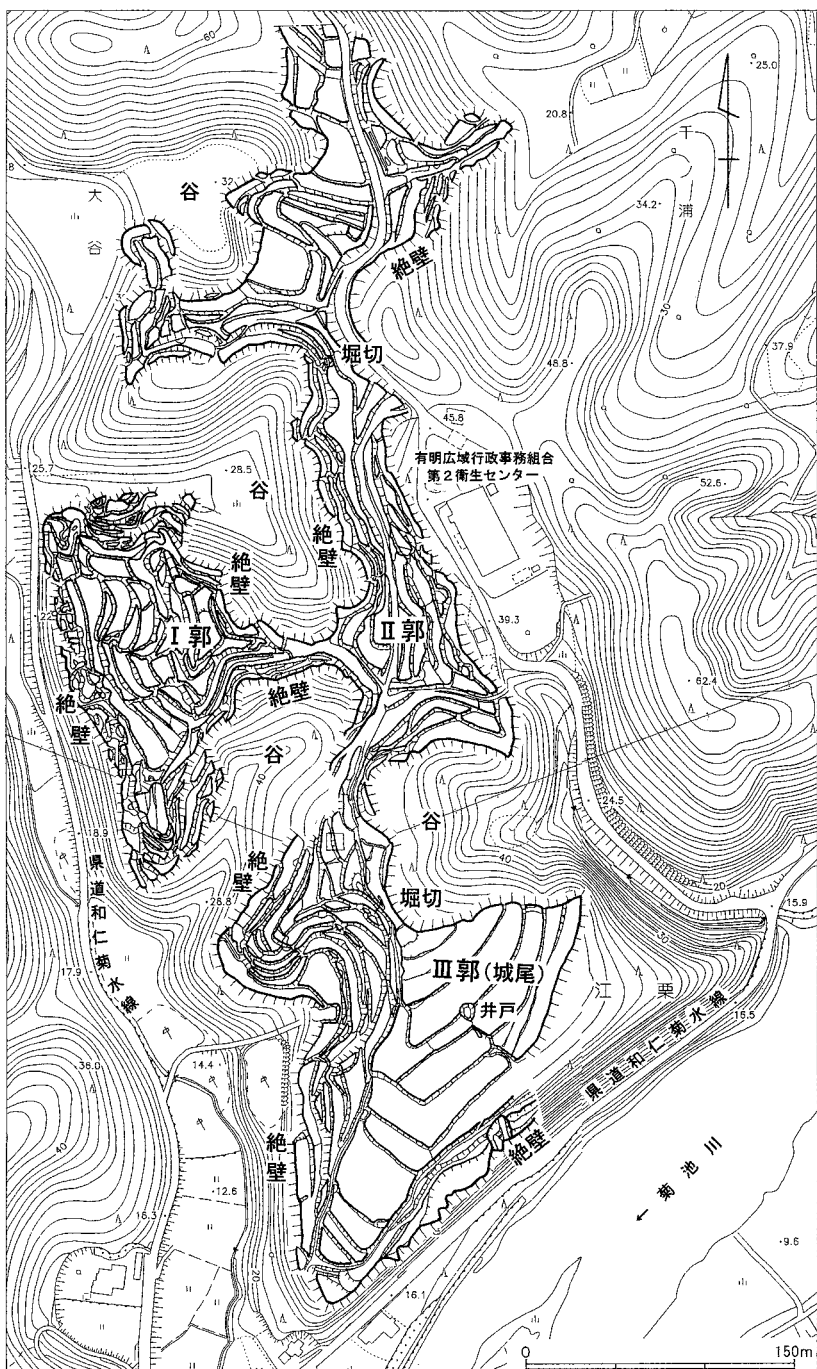
江栗城跡全体縄張り図
