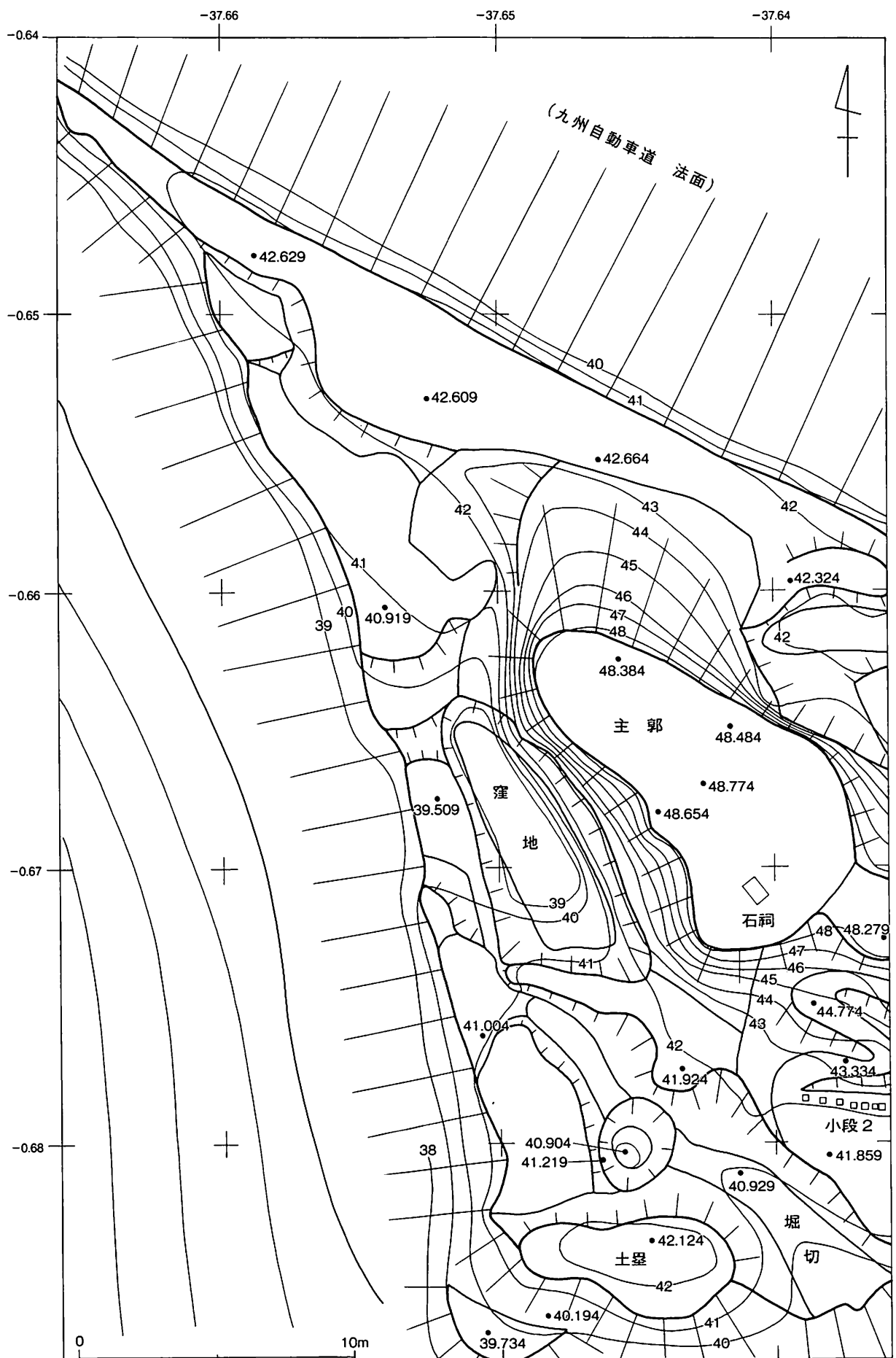
第21図 内田宮山城跡測量図①
