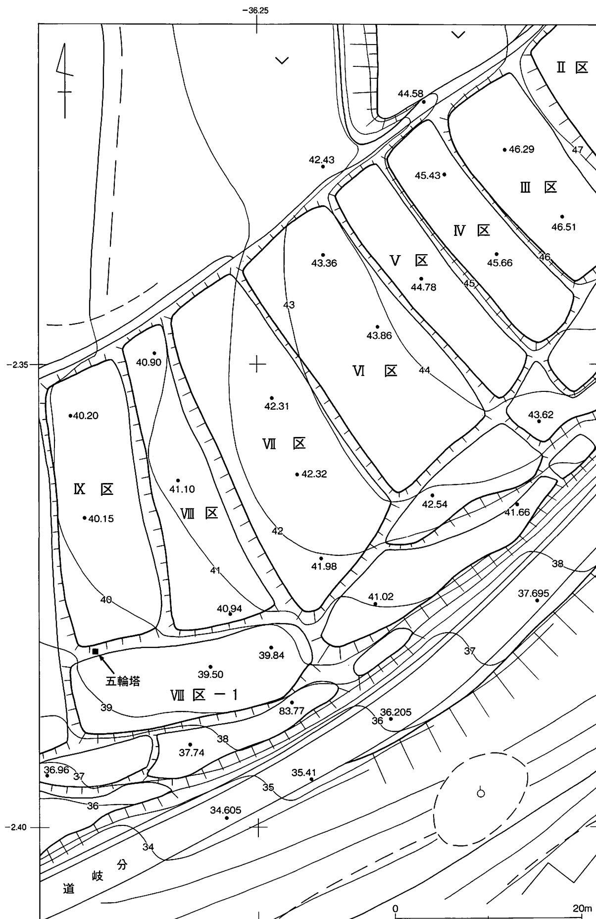
第9図 立石城跡測量図③
