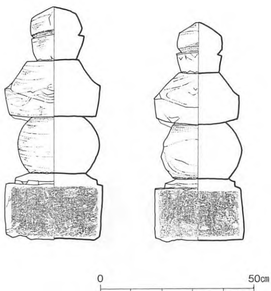
第27図 永正十年銘 五輪塔実測図
