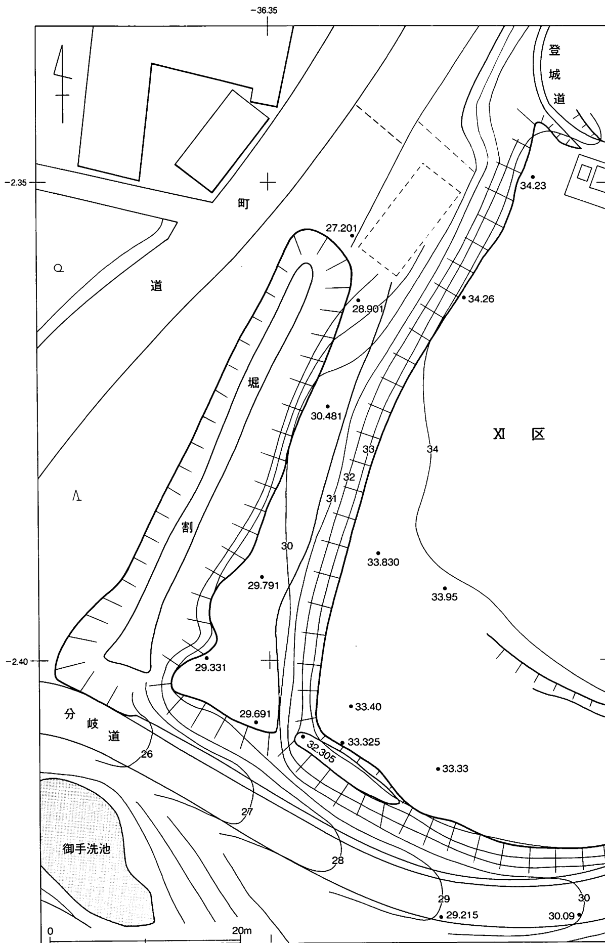
第7図 立石城跡測量図①
