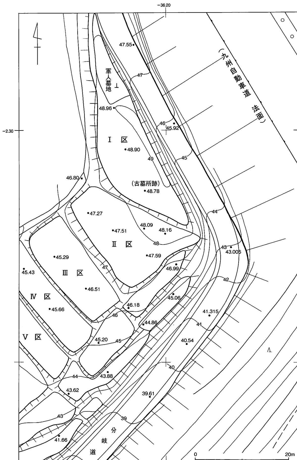
第10図 立石城跡測量図④
