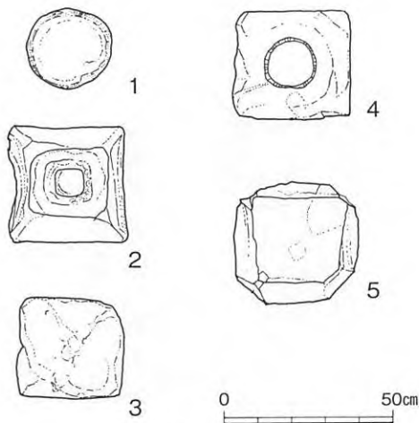
第12図 五輪塔実測図
