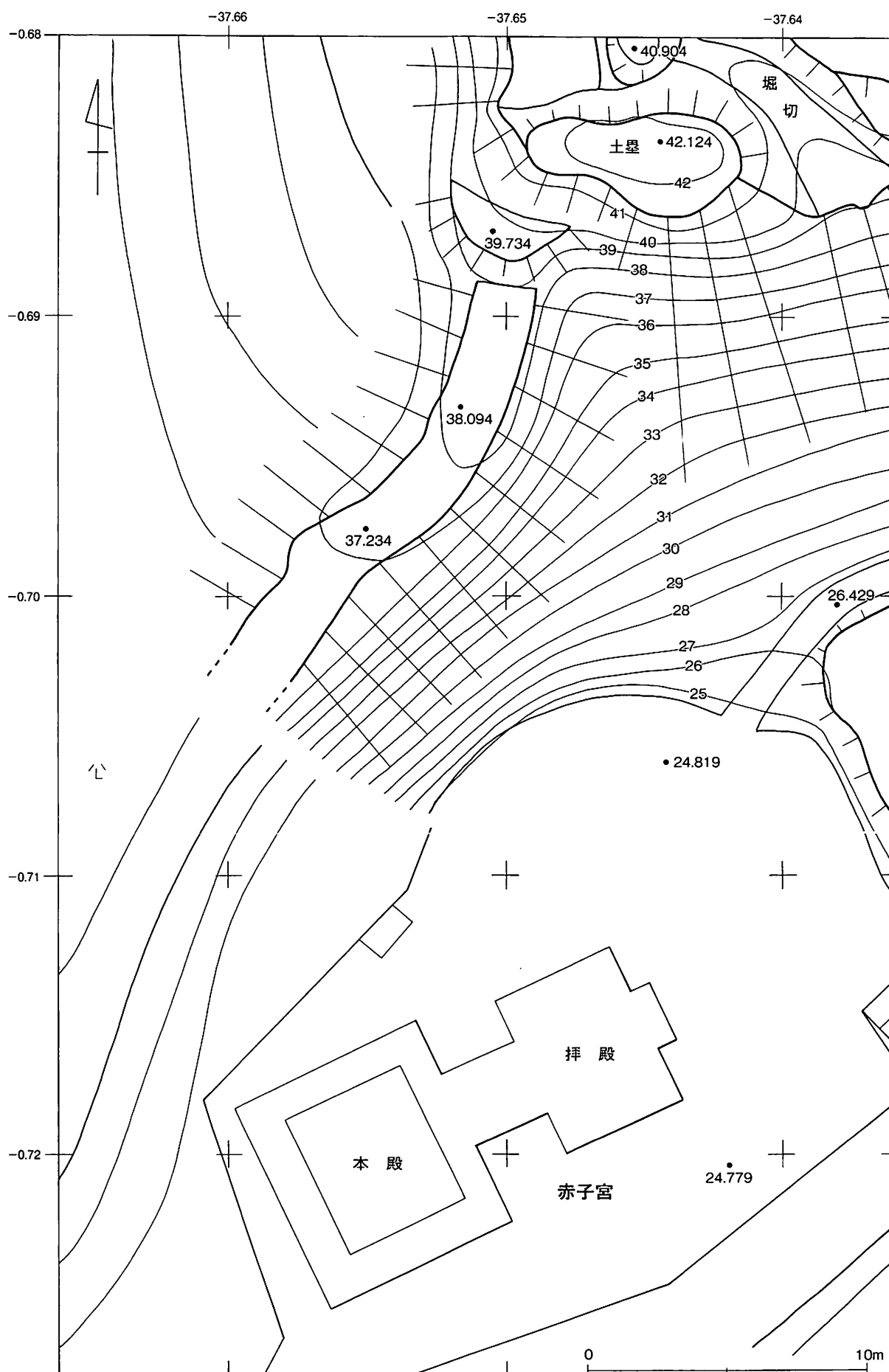
第23図 内田宮山城跡測量図③
