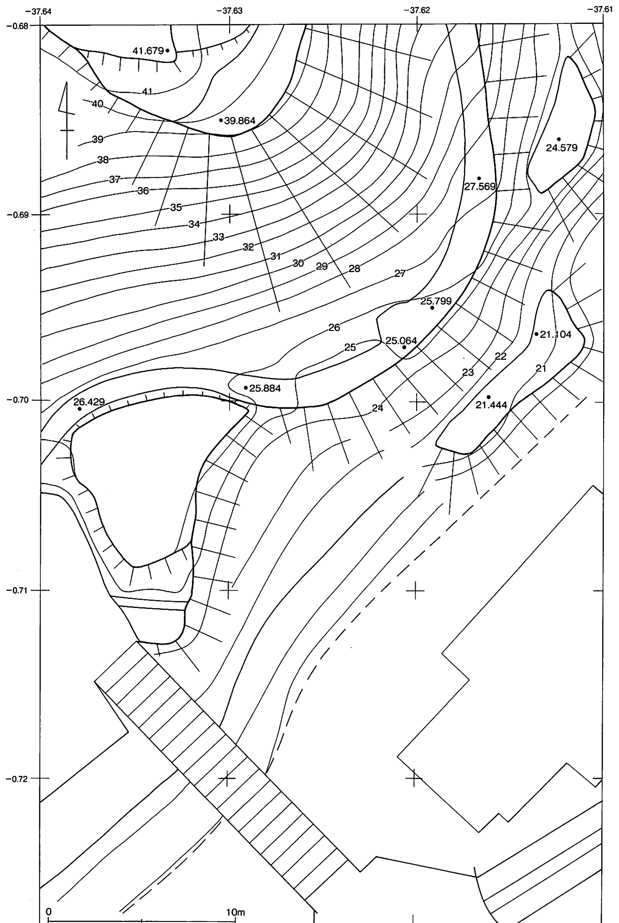
第24図 内田宮山城跡測量図④
