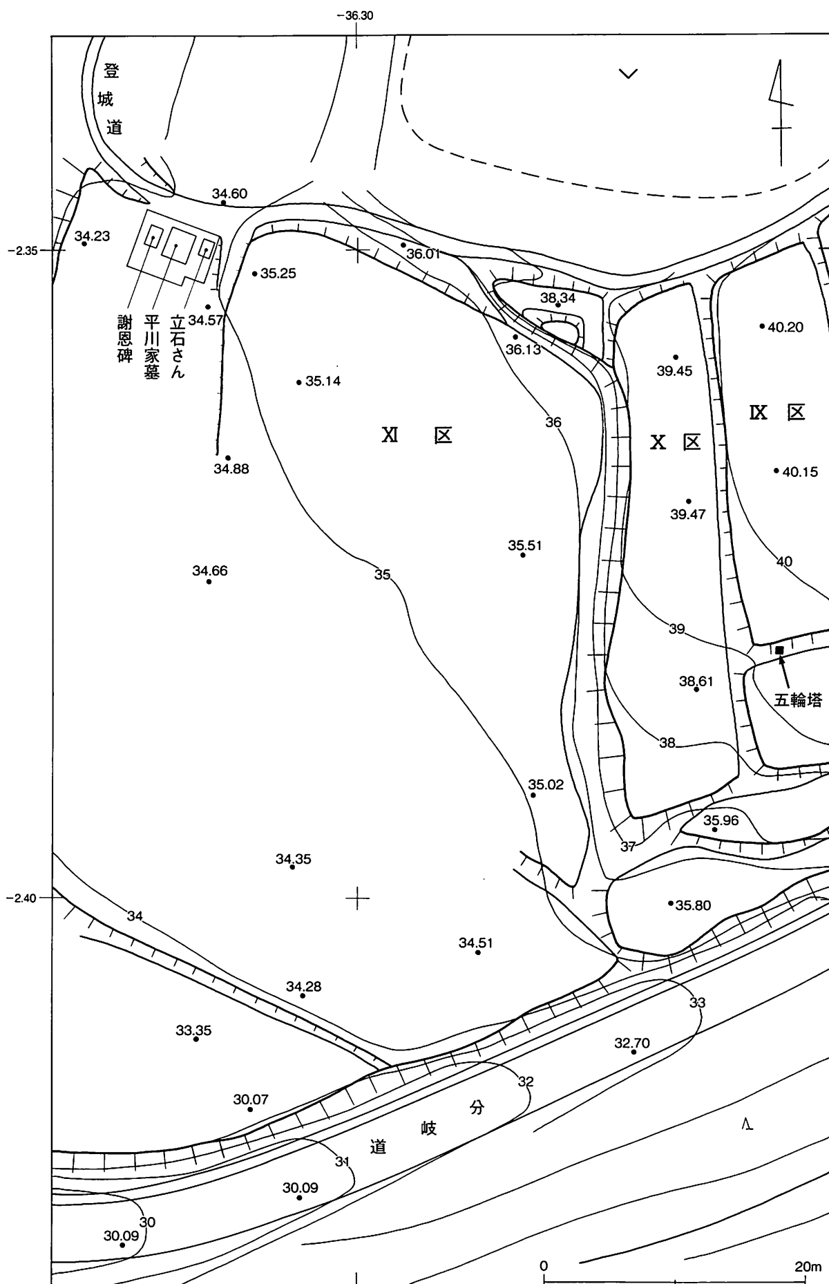
第8図 立石城跡測量図②
