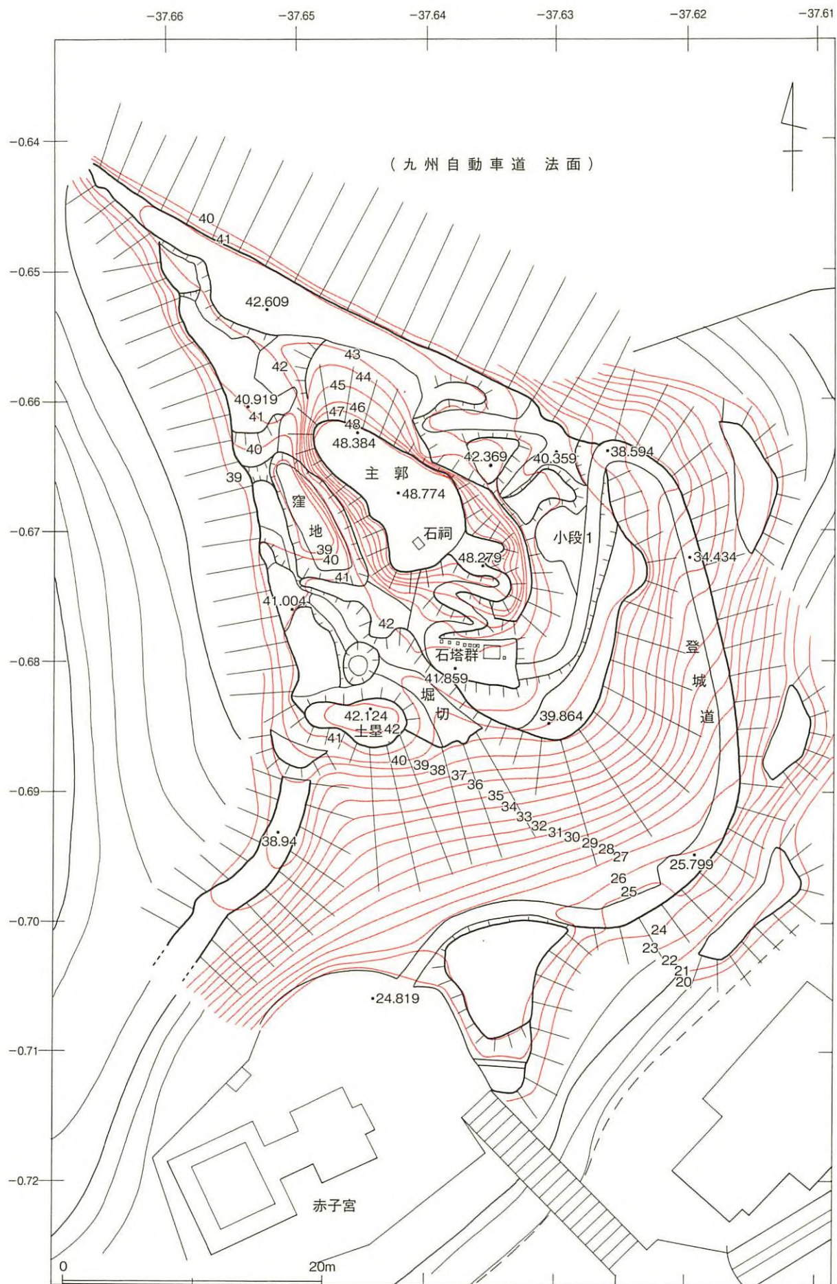
第20図 内田宮山城跡全体測量図
