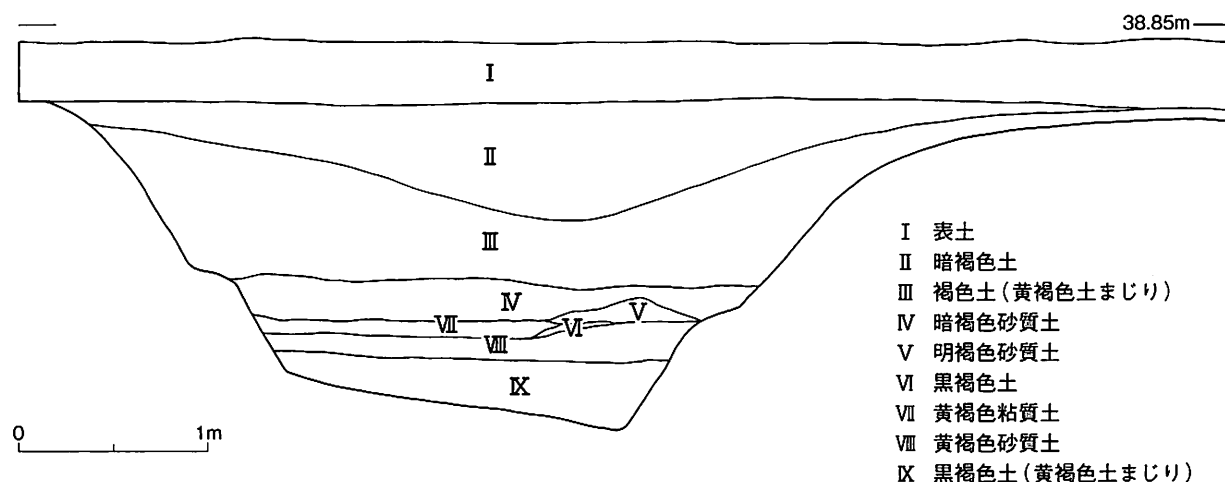
第5図 西側溝状遺構断面実測図
