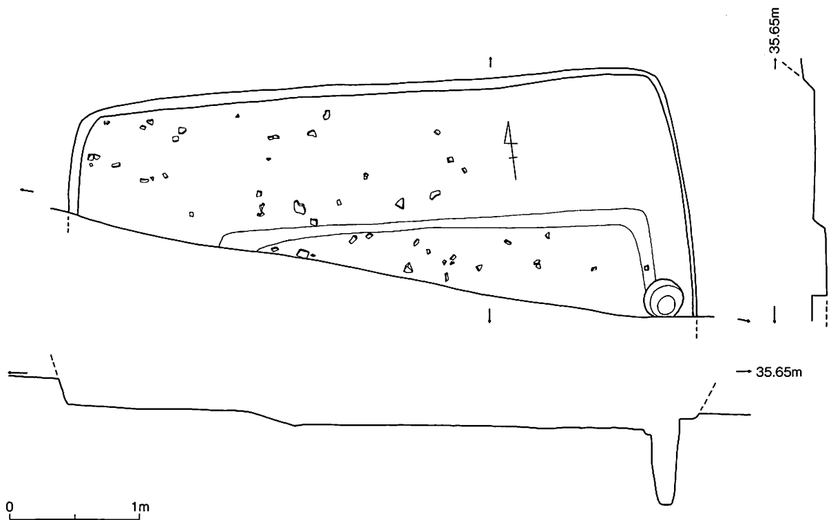
第4図 竪穴式住居実測図
