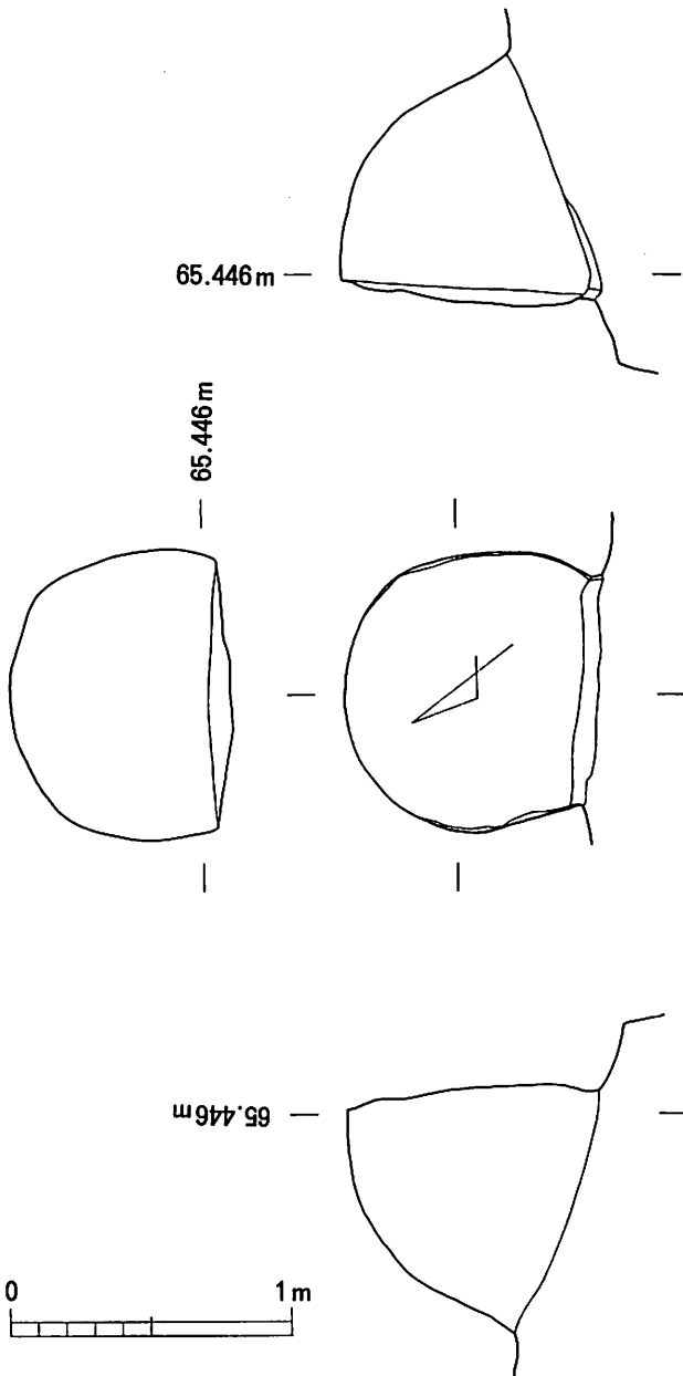
第4図 1号石竈実測図
