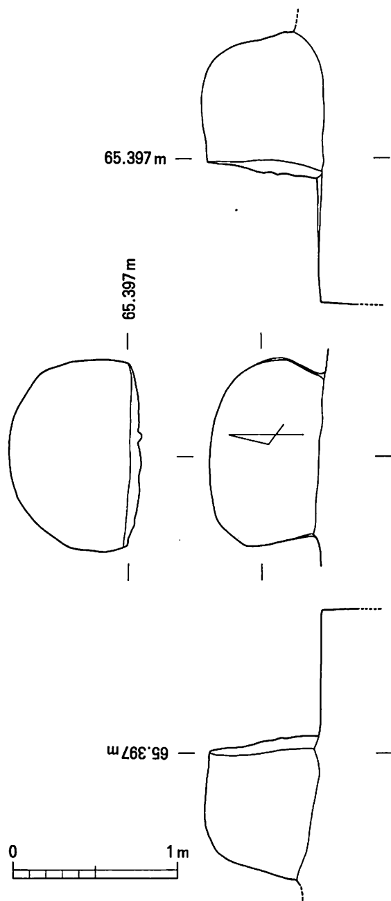
第 5 図 2 号石龕実測図
