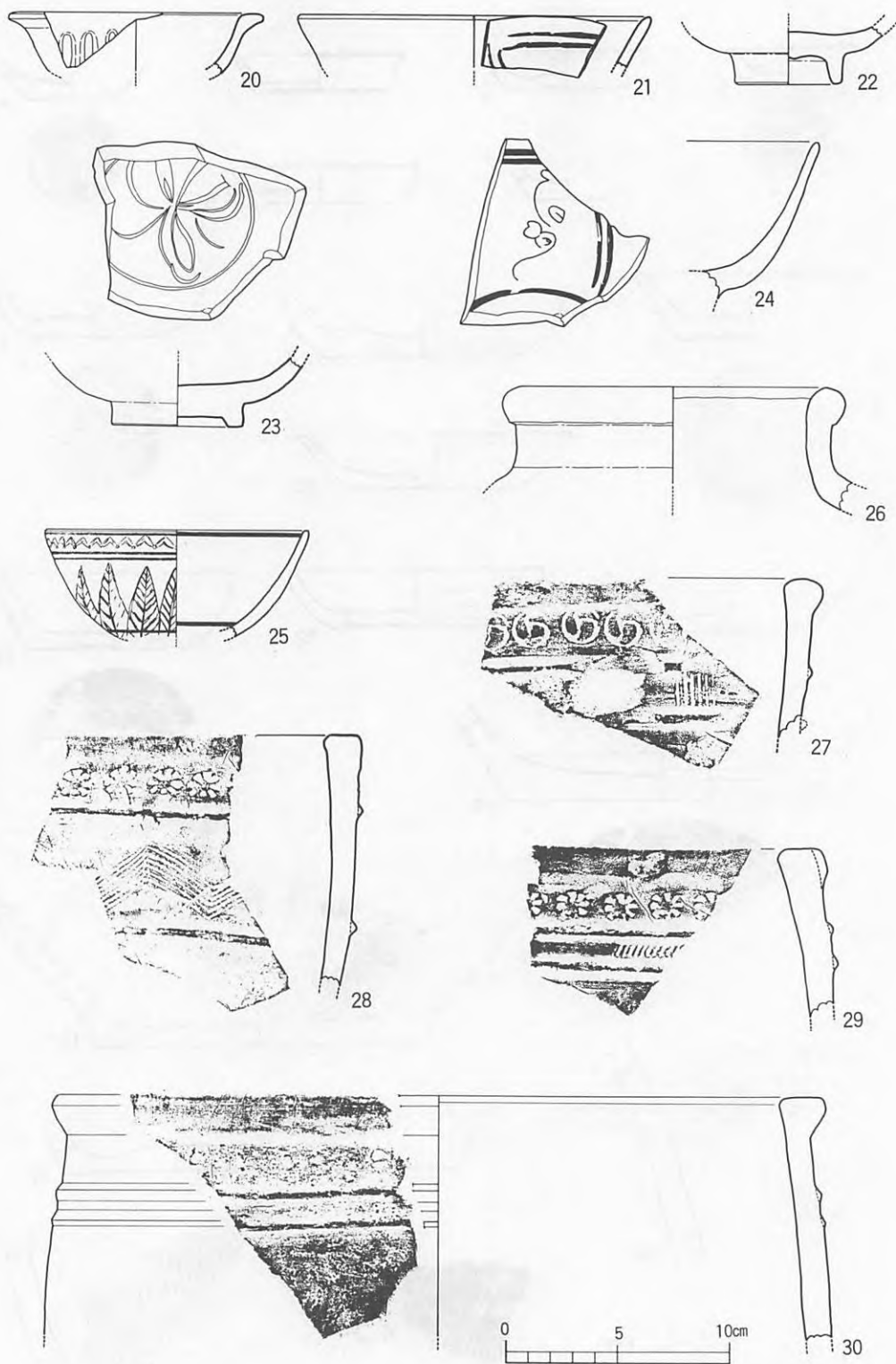
第32図 出土遺物実測図 2
