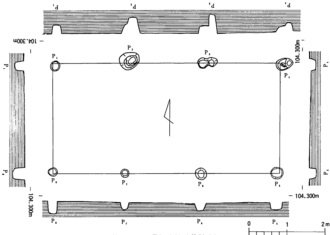
第19図 8号掘立柱建物跡実測図
