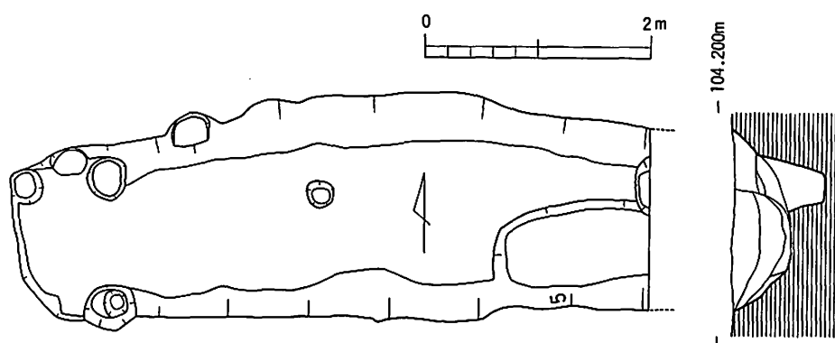
第27図 2号溝実測図
