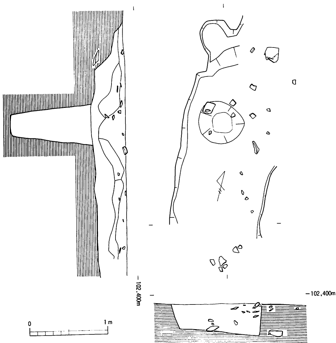
第39図 1号不定形土坑－Ⅱ 実測図
