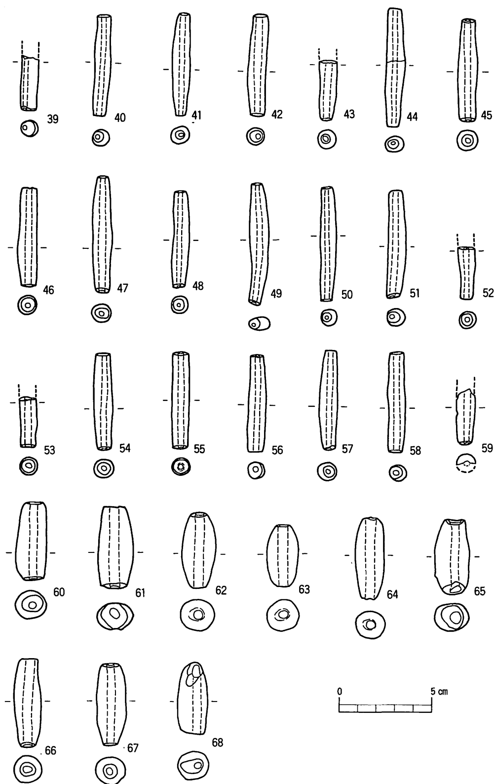
第34図 土錘実測図
