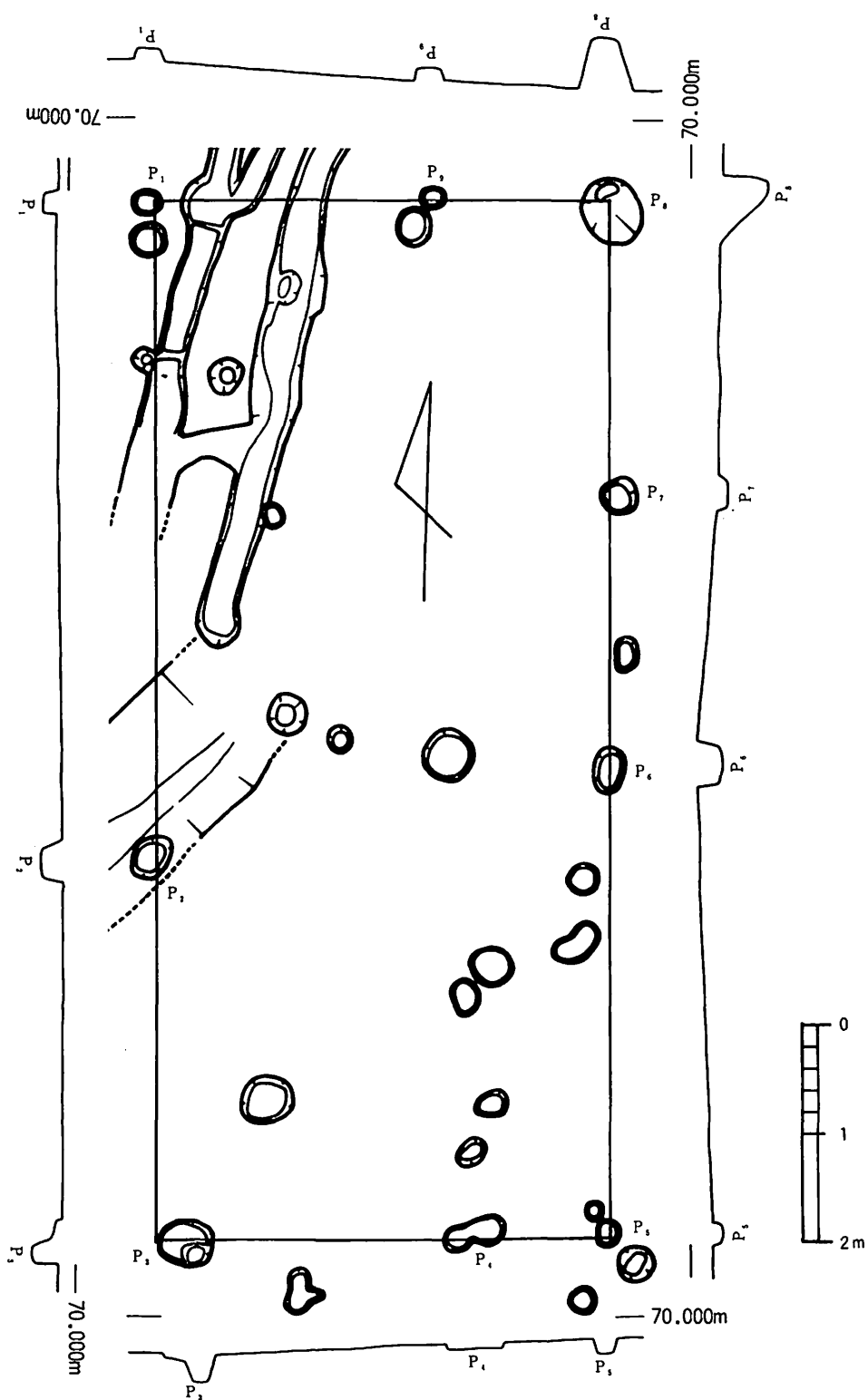
第91図 掘立様建物跡実測図
