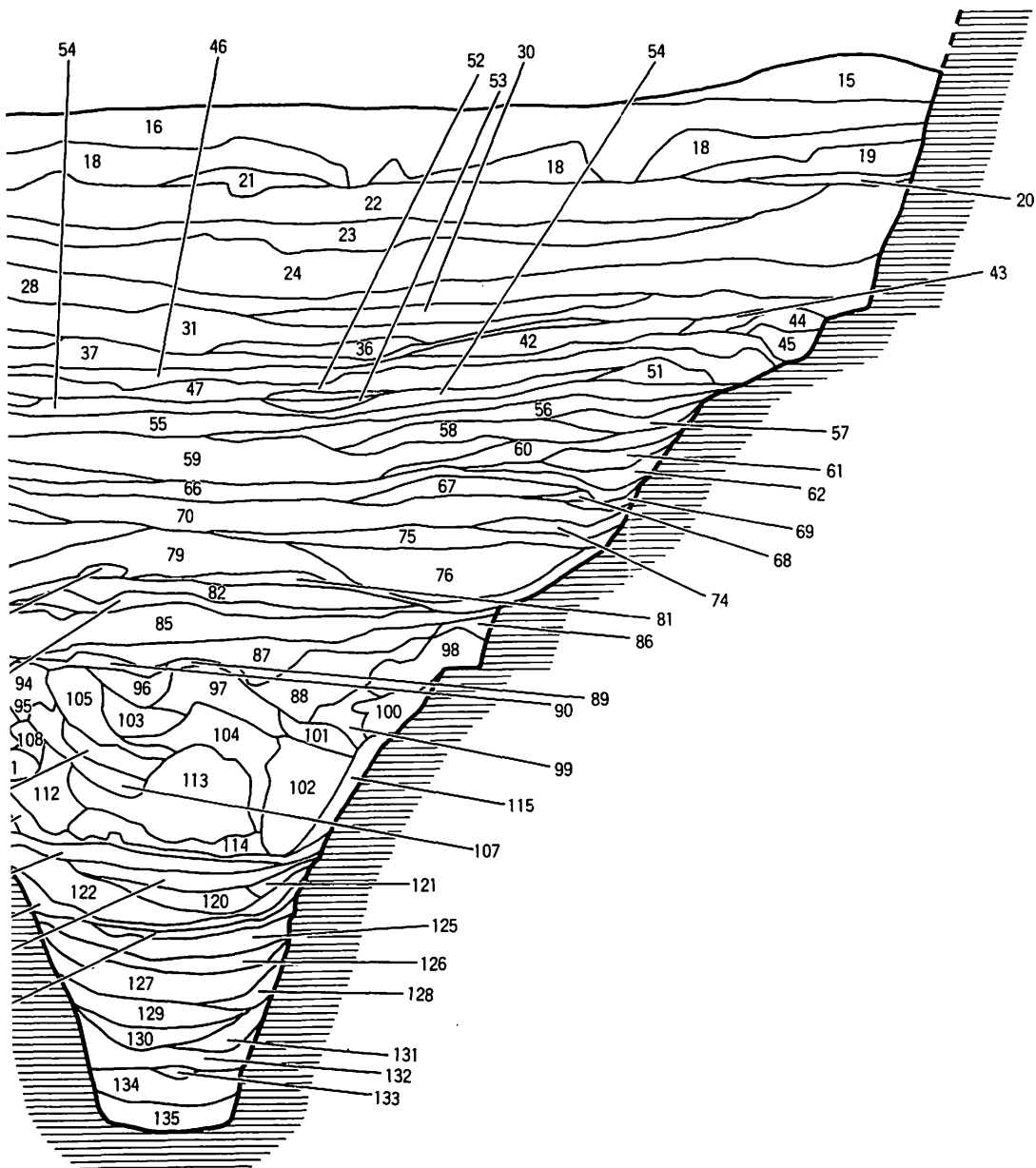
断面实测图
