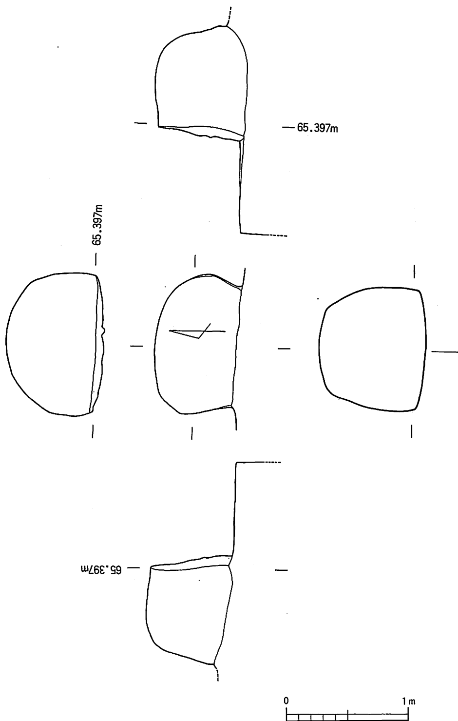
第82図 2号石龕実測図
