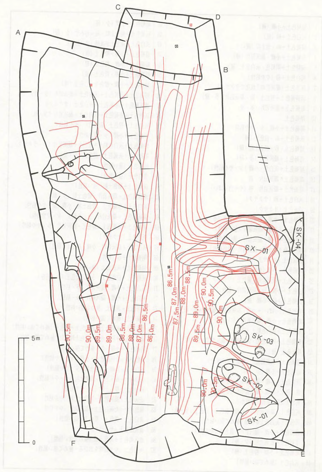
第57図 平成元年度調査 空堀測量図
