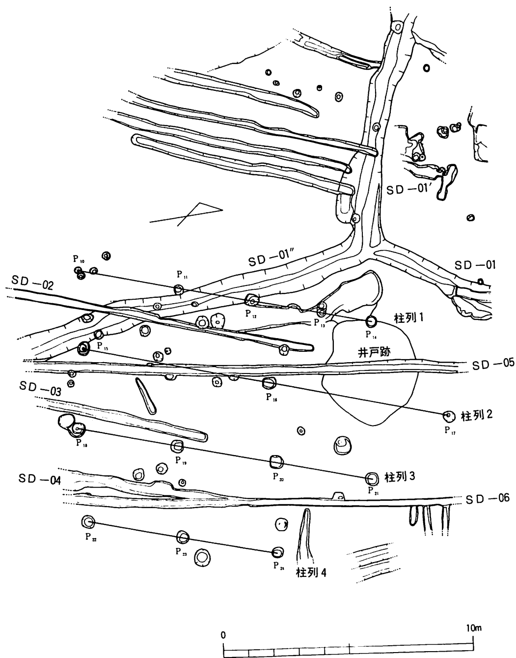
第93図 II区遺構配置図
