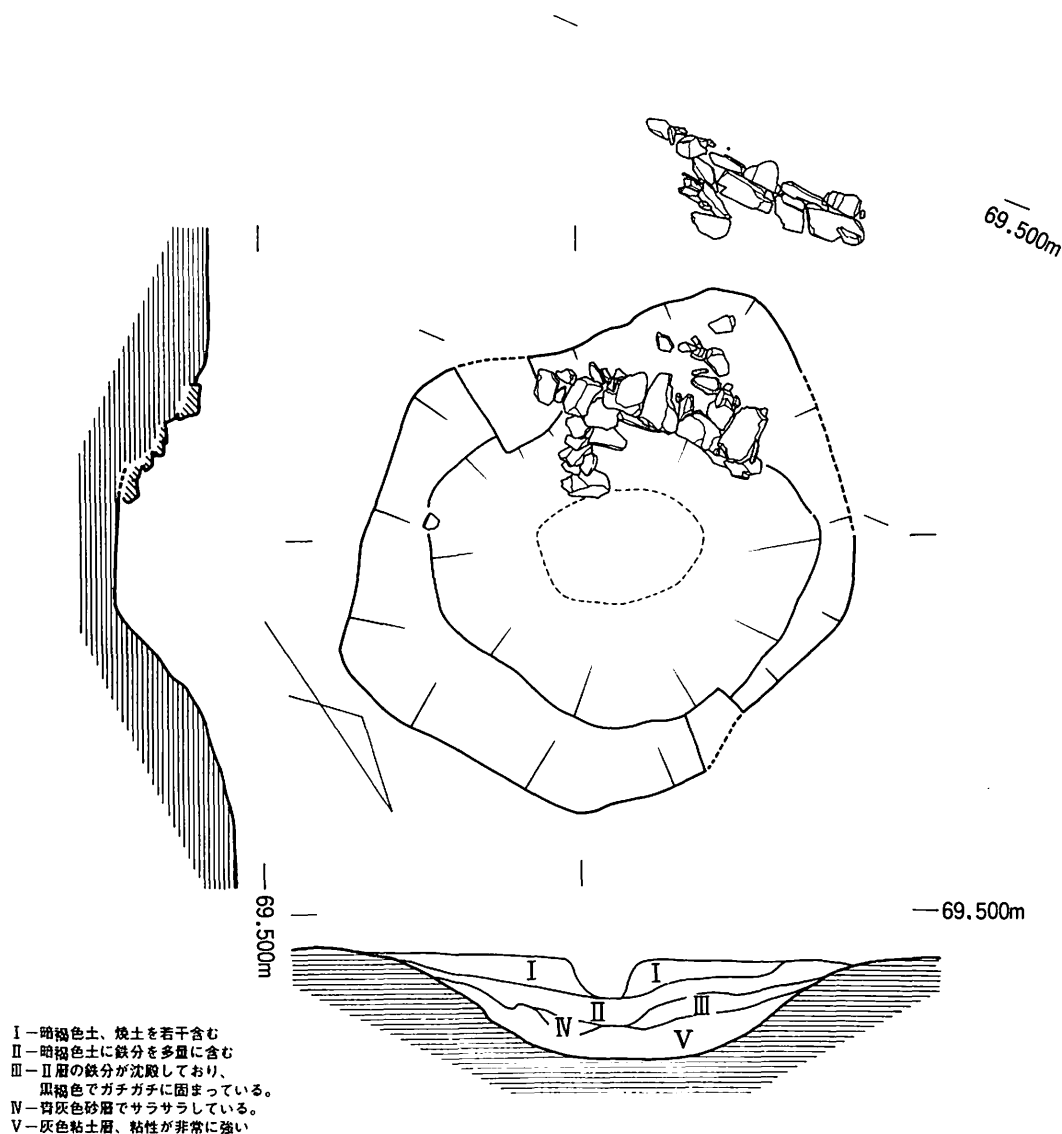
第92図 井戸跡実測図
