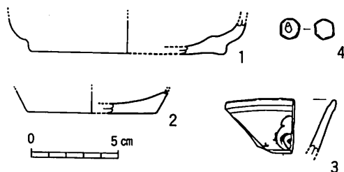
第76図 出土遺物実測図
