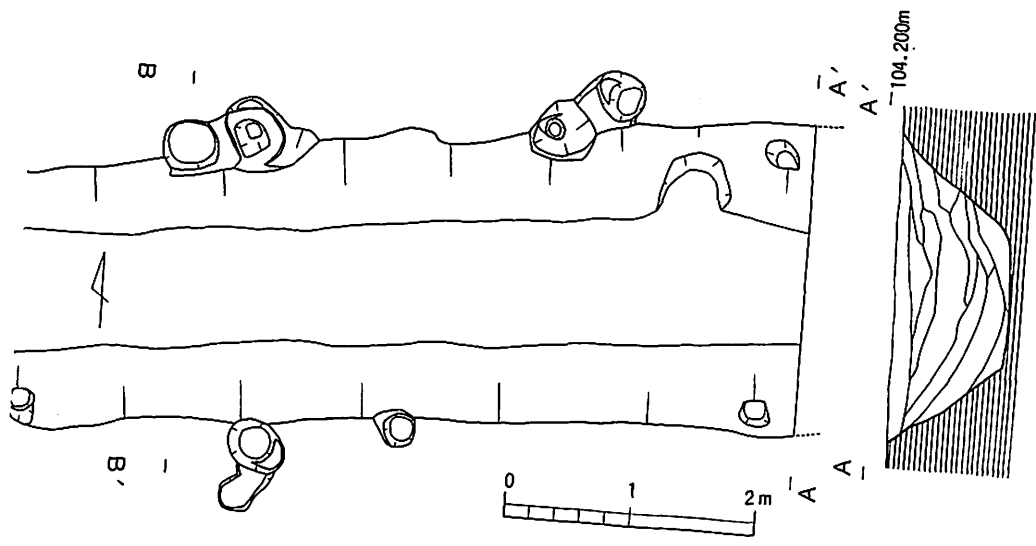
溝実測図
