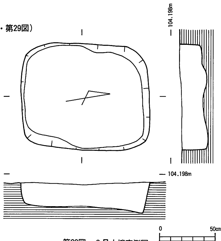
第29図 2号土壇実測図
