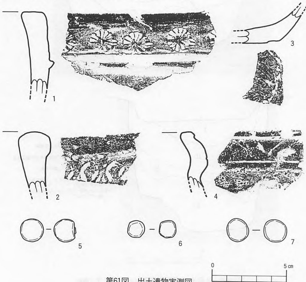
第61図 出土遺物実測図
