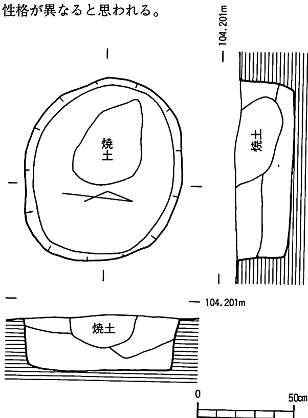
第28図 1号土壌実測図
