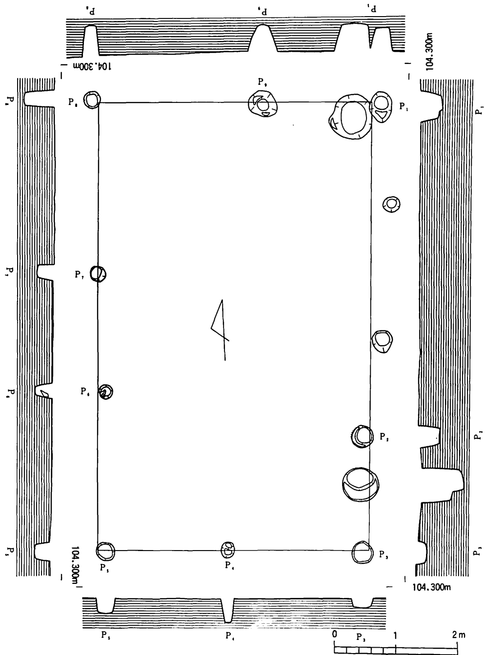
第17図 6号掘立柱建物跡実測図
